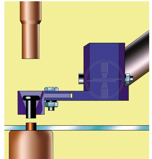
Bolzenzuführeinheit
