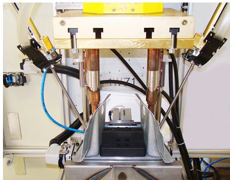
Doppel-Mutternzuführeinheit
