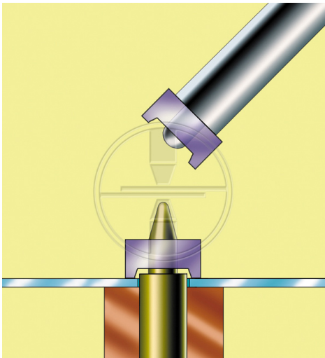
Mutternzuführeinheit
