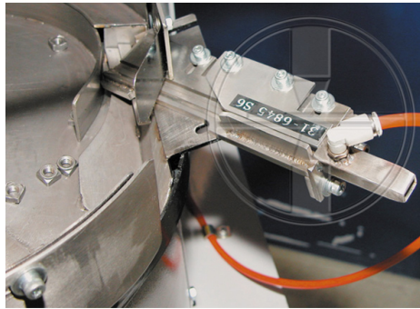
Kassetten-Mutternzuführeinheit
