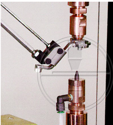
Zuführung oben
