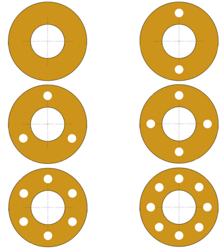
Isolierscheiben
