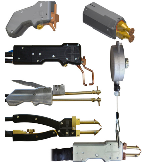
Mikro-Schweißzangen
