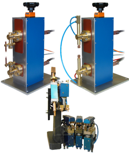
Mikro-Schweißköpfe
