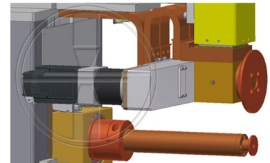
Mikro-Servoantrieb
