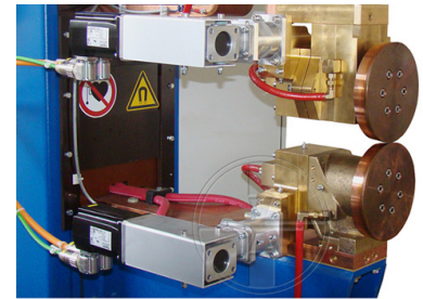
Mikro-Schweißzangen
