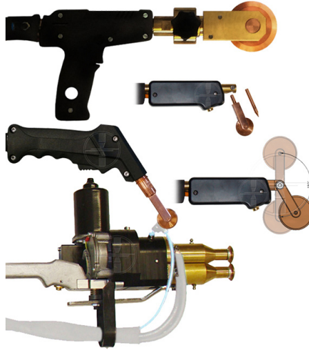
Mikro-Rollnaht
