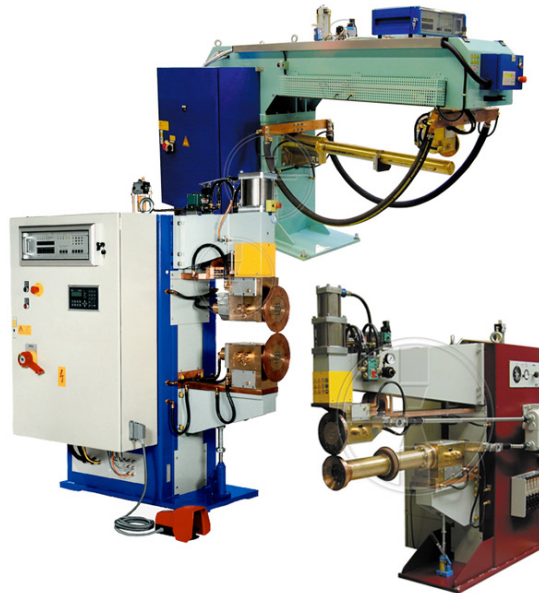
N-Rollenahtschweißmaschinen
