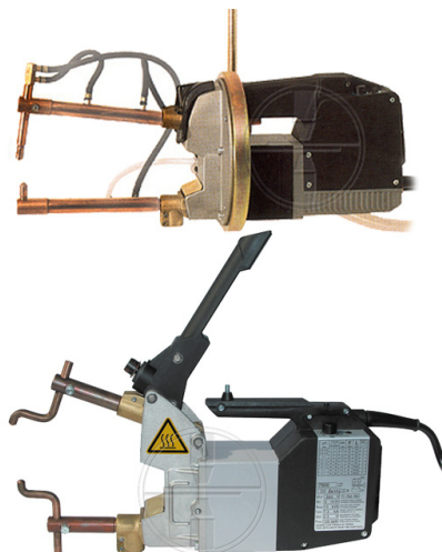
KFZ-Punktschweißzangen
