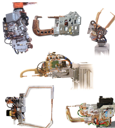
Roboterschweißzangen
