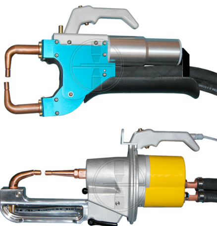
Kabel-Punktschweißzangen
