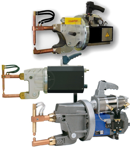
X-Punktschweißzangen
