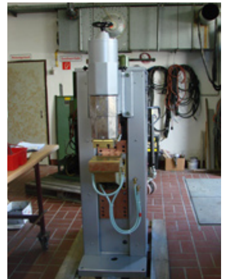
DALEX BSM 14-2-AC 2-Phasen-Wechselstrom-Buckel-Schweißmaschine
